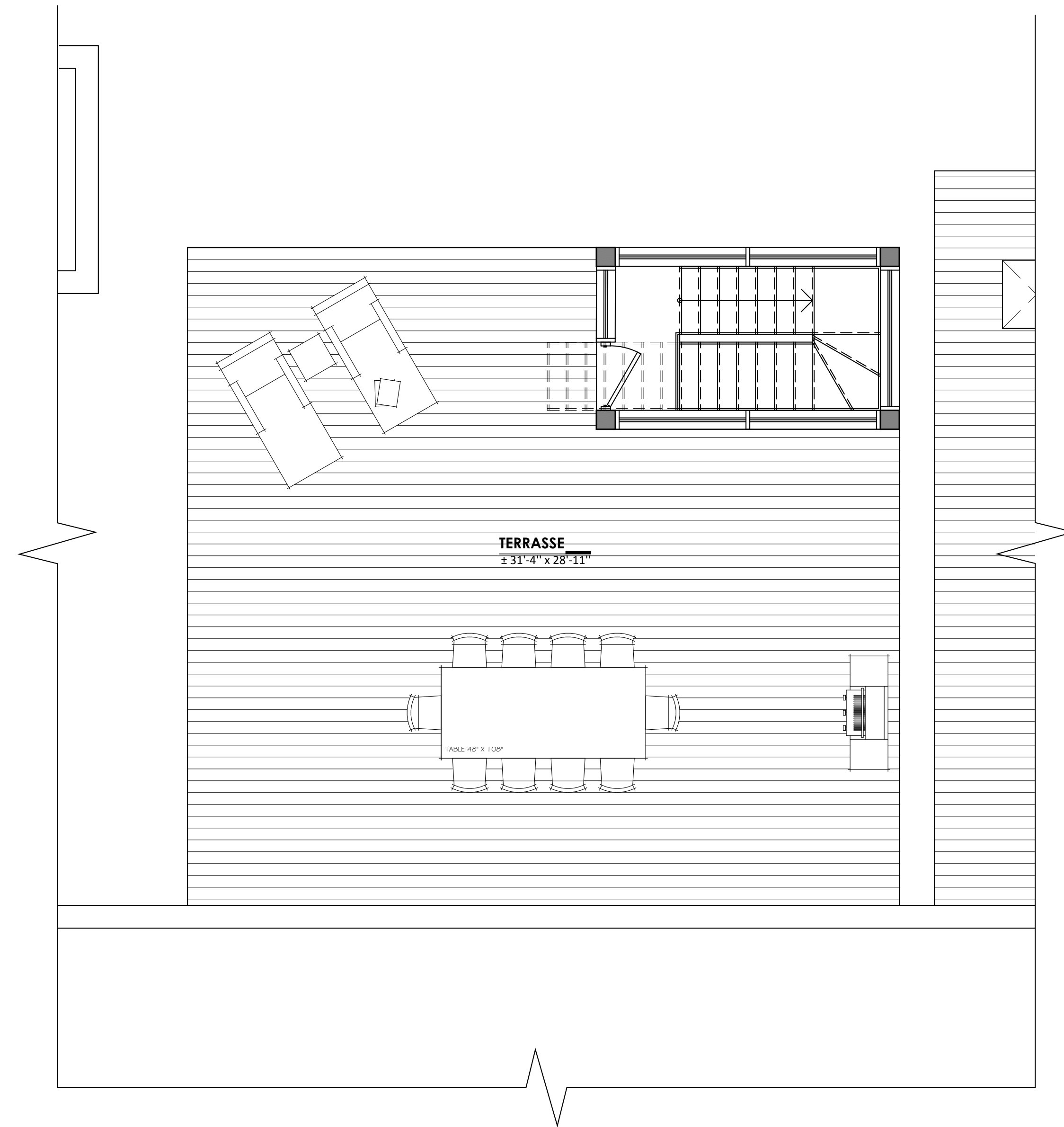
ÉCHELLE: 1/4" = 1'-0"
