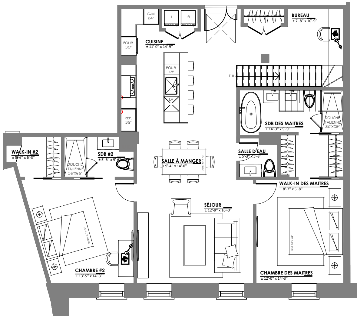
ÉCHELLE: 1/8" = 1'-0"
